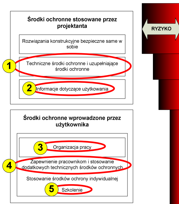
Rys.2 Umiejscowienie roli osłon w procesie redukcji ryzyka na podstawie normy PN-EN ISO 12100-1. Na rysunku numerami od 1 do 5 oznaczono elementy mające związek z osłonami lub ich użytkowaniem (wyjaśnienie w tekście).
